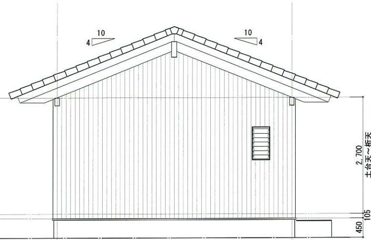
東立面図 S=1:60
