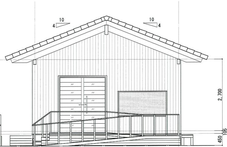
西立面図 S=1:60
