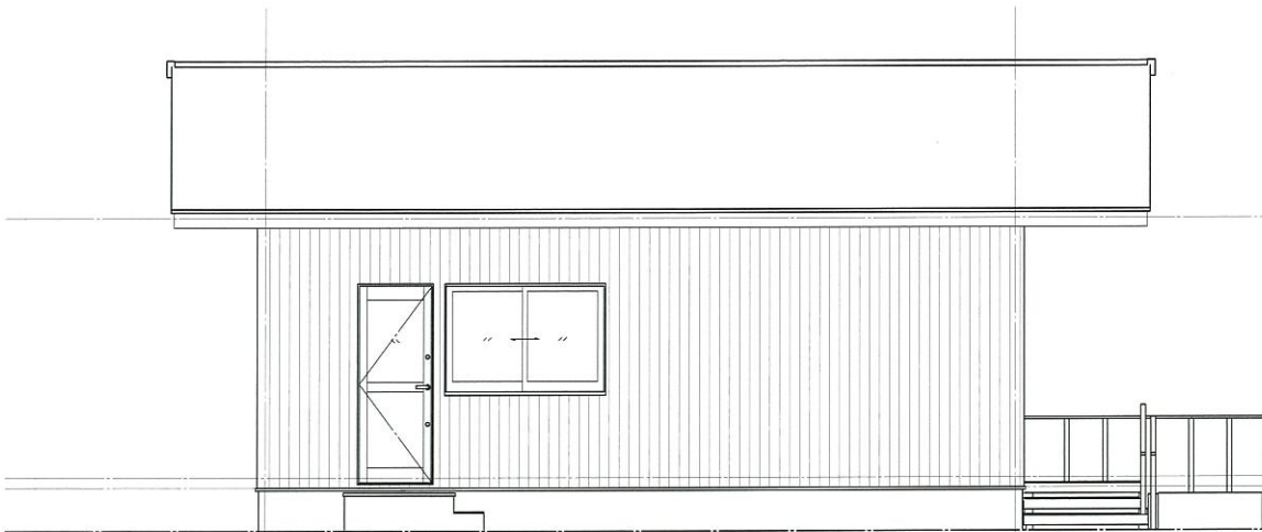
北立面図 S=1:60
